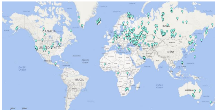
Рис. 10. Описанные выходы водорода с концентрацией >10% (по данным >330 статей и >20 книг) [9].
